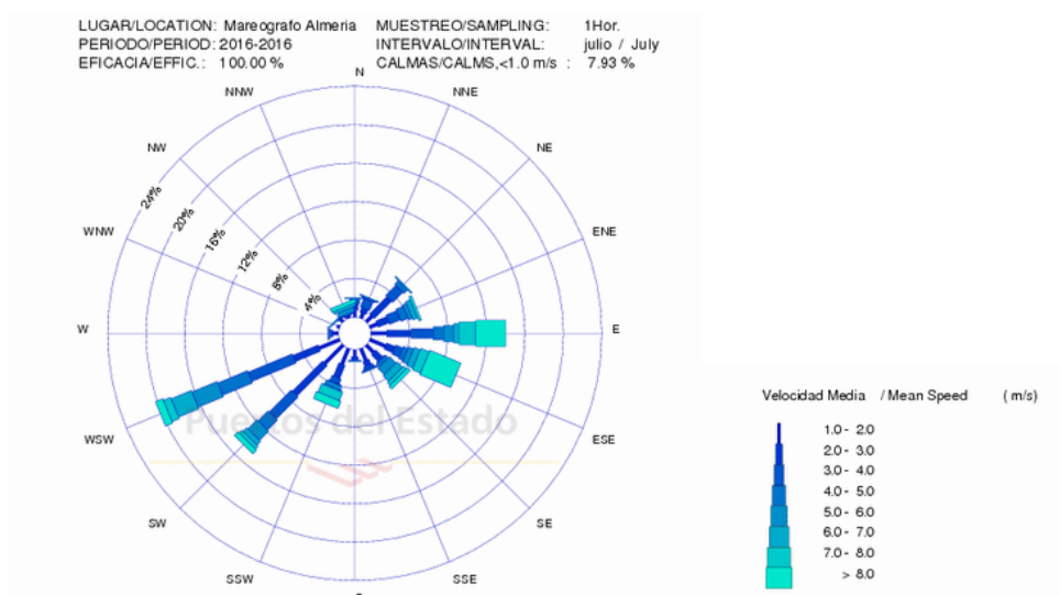
Figura 2. Rosa de los vientos correspondiente al mes de julio de 2016 (mareógrafo de Almería, fuente: Puertos del Estado).
