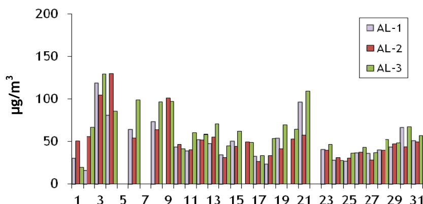
Figura 1. Evolución temporal de la concentración de partículas en suspensión en las estaciones de muestreo situadas en el Puerto de Almería. Julio 2016.
