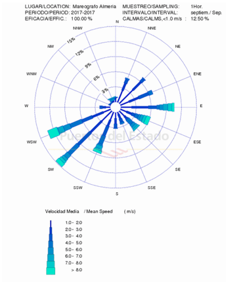
Figura 2. Rosa de los vientos correspondiente al mes de septiembre de 2017 (mareógrafo de Almería, fuente: Puertos del Estado).
