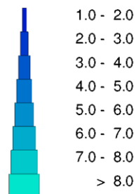
Figura 2. Rosa de los vientos correspondiente al mes de octubre de 2019 (mareógrafo de Almería, fuente: Puertos del Estado).
