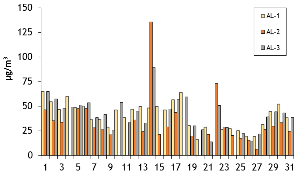
Figura 1. Evolución temporal de la concentración de partículas en suspensión en las estaciones de muestreo situadas en el Puerto de Almería. Octubre 2019.
