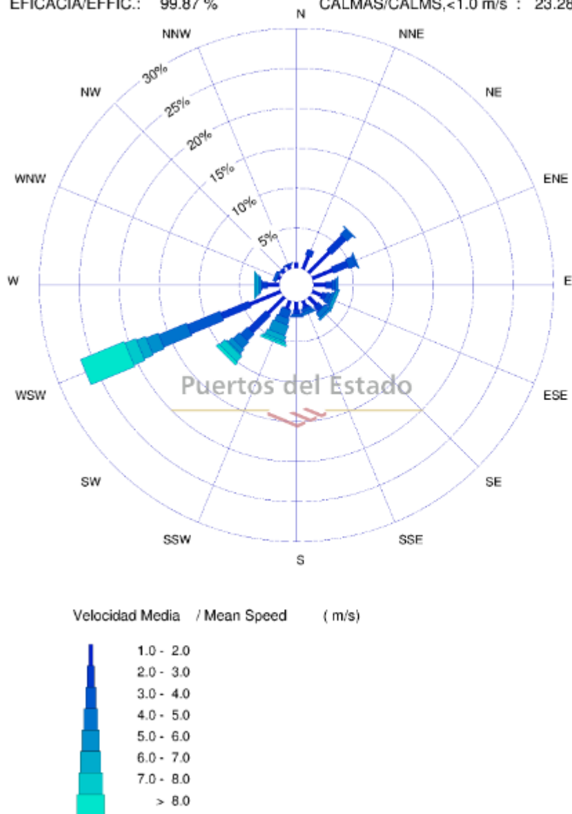
Figura 2. Rosa de los vientos correspondiente al mes de octubre de 2020 (Mareógrafo de Almería, fuente: Puertos del Estado).
