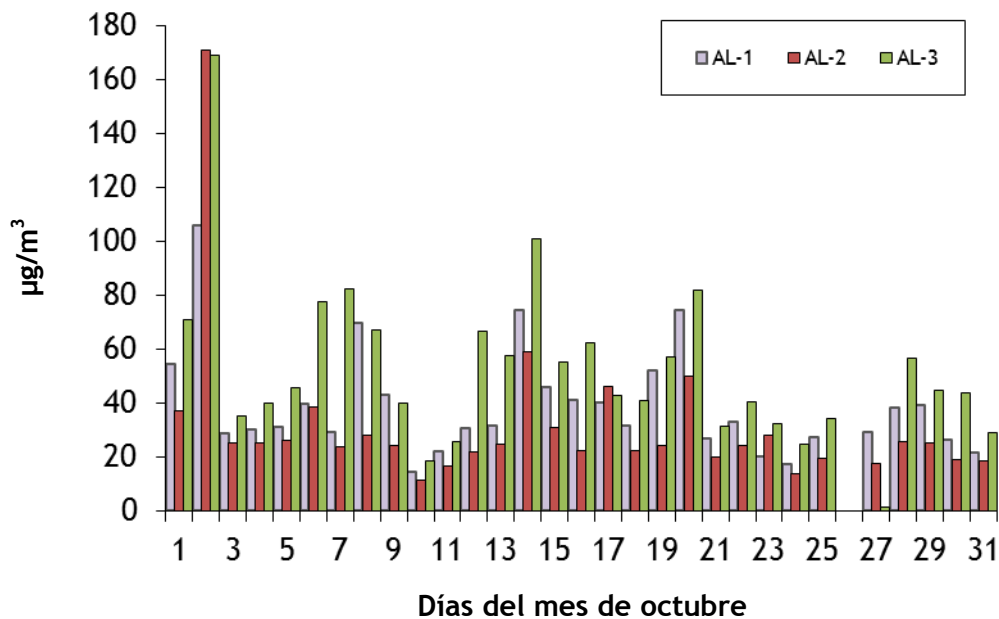
Figura 1. Evolución temporal de la concentración de partículas en suspensión en las estaciones de muestreo situadas en el Puerto de Almería. Octubre 2020
