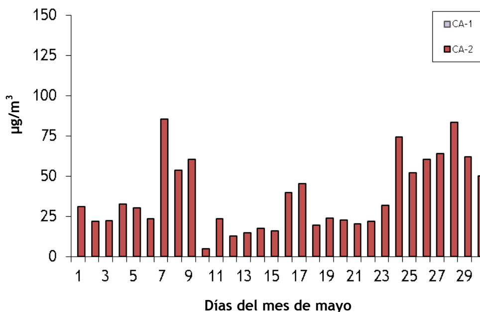
Figura 1. Evolución temporal de la concentración de partículas PM 10 en las estaciones de muestreo situadas en el Puerto de Carboneras. Mayo 2020
