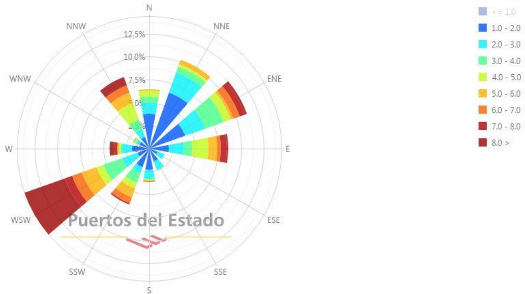
Figura 2. Rosa de los vientos correspondiente al mes de diciembre de 2021 (Mareógrafo de Almería, fuente: Puertos del Estado).
