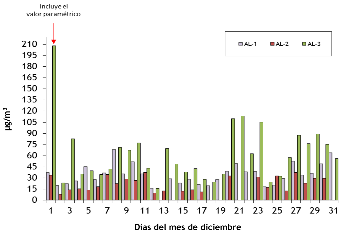
Figura 1. Evolución temporal de la concentración de partículas en suspensión en las estaciones de muestreo situadas en el Puerto de Almería. Diciembre 2021.
