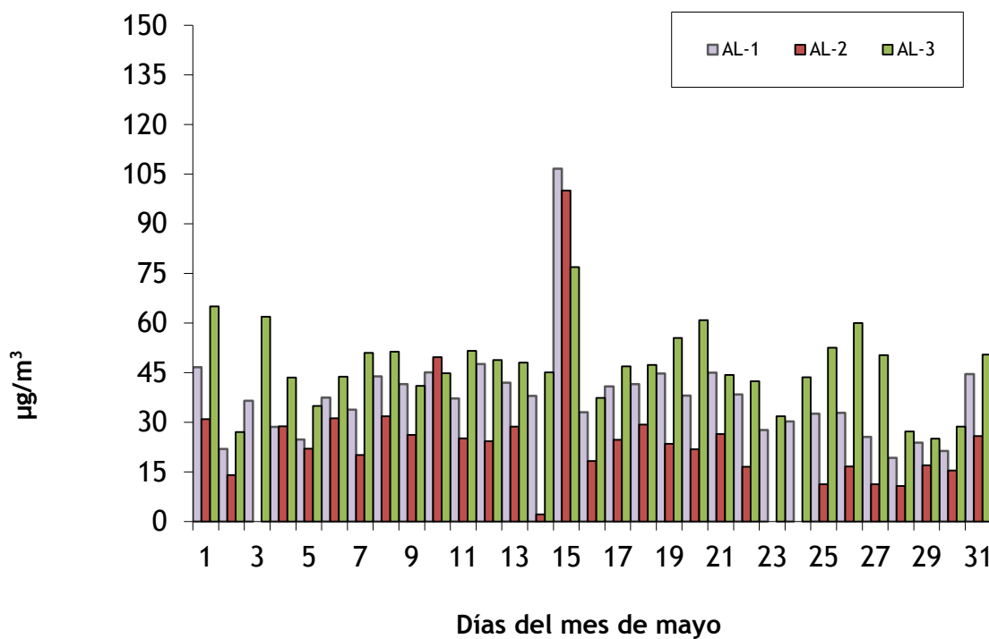
Figura 1. Evolución temporal de la concentración de partículas en suspensión en las estaciones de muestreo situadas en el Puerto de Almería. Mayo 2021.
