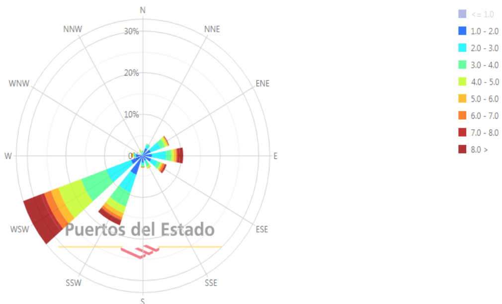
Figura 2. Rosa de los vientos correspondiente al mes de julio de 2021 (Mareógrafo de Almería, fuente: Puertos del Estado).
