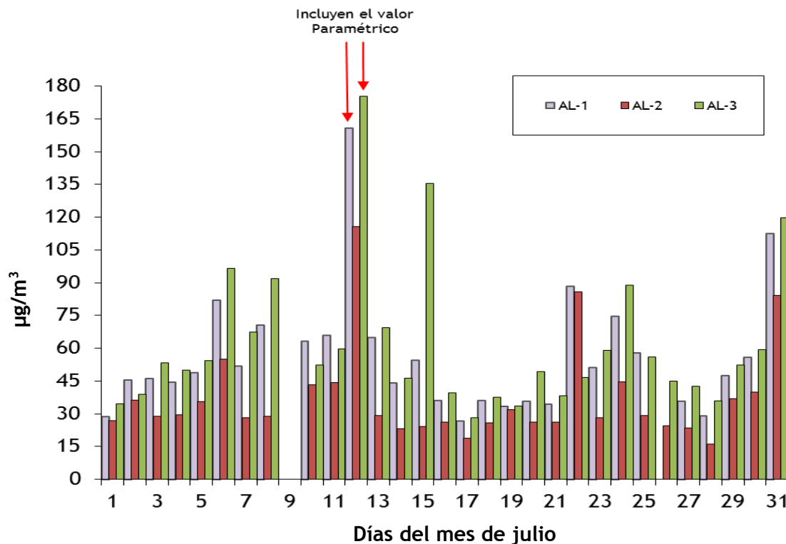
Figura 1. Evolución temporal de la concentración de partículas en suspensión en las estaciones de muestreo situadas en el Puerto de Almería. Julio 2021. El día 9 no se toman muestras en ninguna estación y el día 26 en AL-1.
