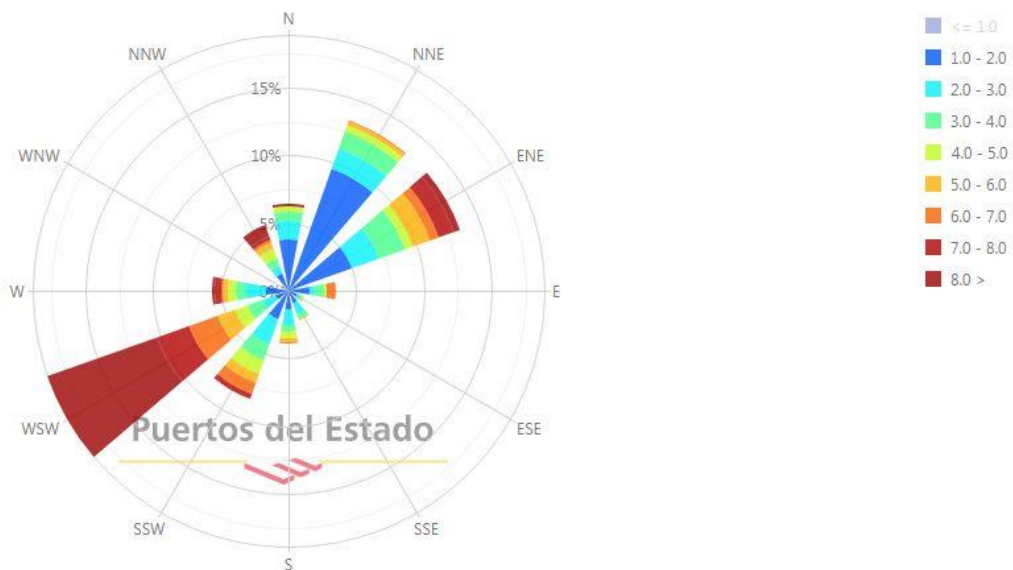
Figura 2. Rosa de los vientos correspondiente al mes de noviembre de 2021 (Mareógrafo de Almería, fuente: Puertos del Estado).
