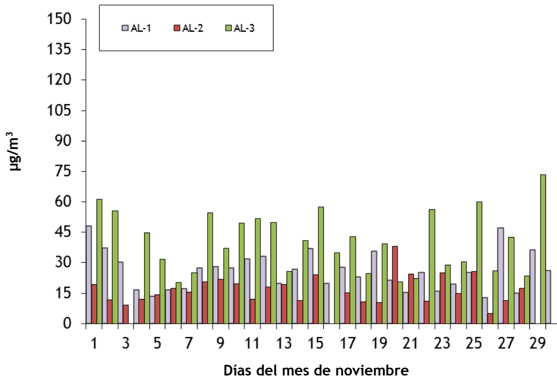
Figura 1. Evolución temporal de la concentración de partículas en suspensión en las estaciones de muestreo situadas en el Puerto de Almería. Noviembre 2021. No se tienen datos de los días 1, 2 y 18 en la estación AL-2, y de los días 3 y 30 de la estación AL-3.
