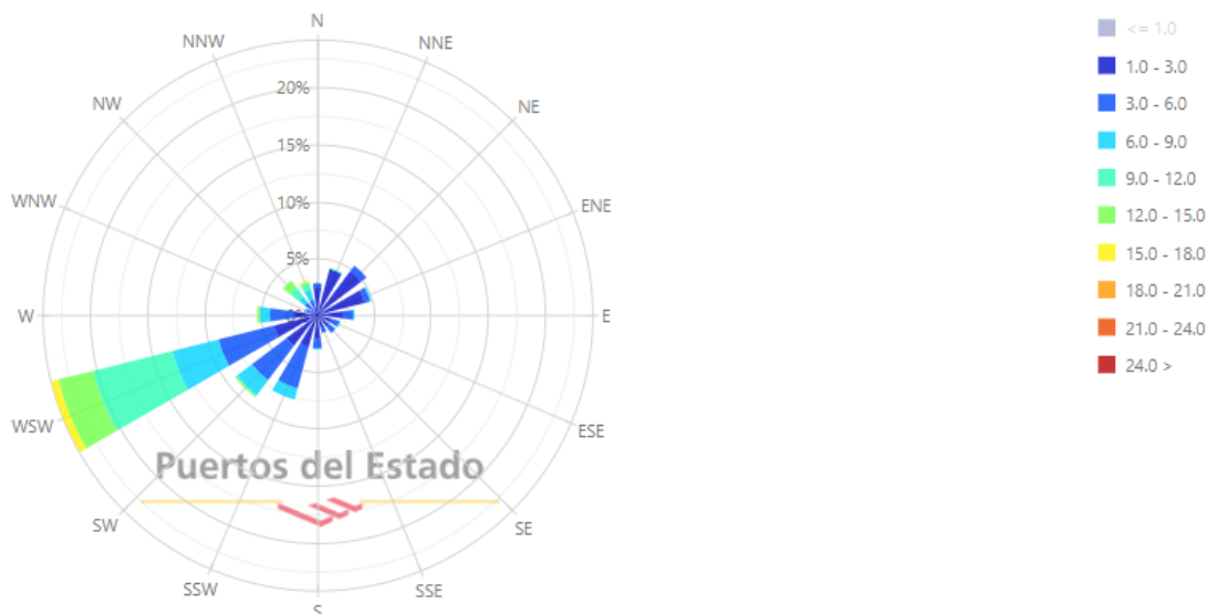
Figura 2. Rosa de los vientos correspondiente al mes de Febrero de 2024 (Mareógrafo de Almería, fuente: Puertos del Estado).
