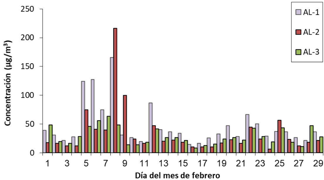
Figura 1. Evolución temporal de la concentración de partículas en suspensión en las estaciones de muestreo situadas en el Puerto de Almería. Febrero 2024.
