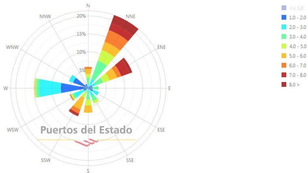
Rosa de Velocidad Media (m/s) para Viento - Mareógrafo de Carboneras Periodo: Septiembre (2021 - 2021) - Eficacia: 57.08%
