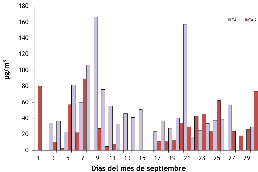
Figura 1. Evolución temporal de la concentración de partículas PM 10 en las estaciones de muestreo situadas en el Puerto de Carboneras. Septiembre 2021. De CA-1 no se tienen resultados los días 1, 2, 16, 28 y 29 de septiembre. Del CA-2 no se tienen resultados de los días 2, 8, del 12 al 16 y el 26 de septiembre.
